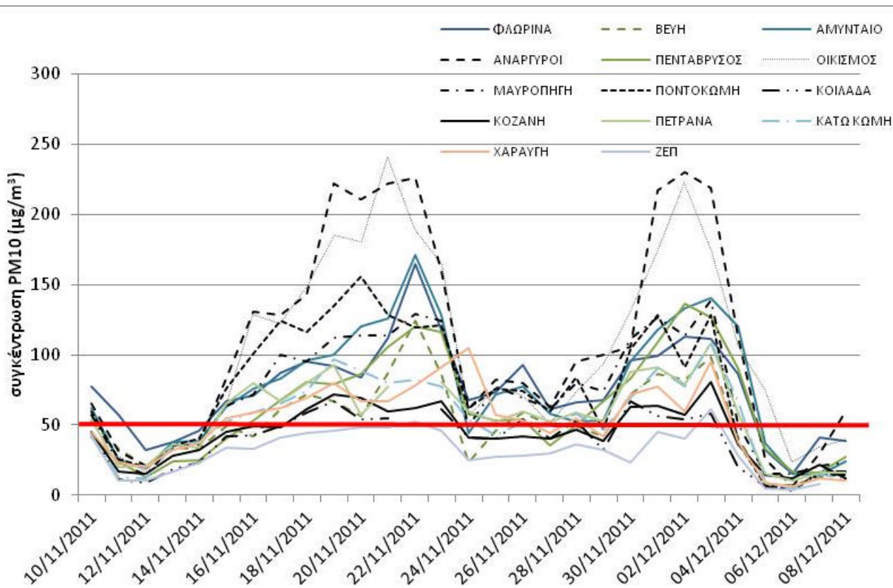
ΣΧΗΜΑ Π.2. Μέσες ημερήσιες συγκεντρώσεις ΑΣ10 σε διάφορες θέσεις μέτρησης την περίοδο από 10/11/2011 έως 08/12/2011. Η κόκκινη γραμμή δείχνει τη μέση ημερήσια οριακή τιμή των 50 µg/m 3 .
